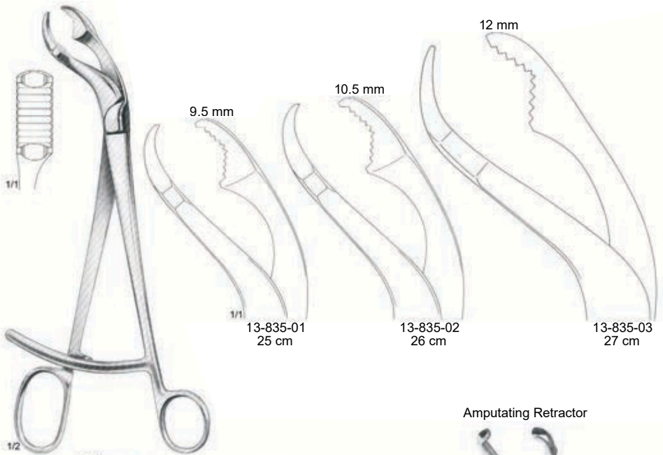
Verbrugge 13-835-01 - 13-835-03
